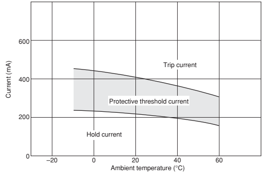
PTGL12AR150H8B72B0
