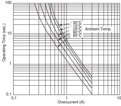
PTGL07AS5R6K4B51B0
