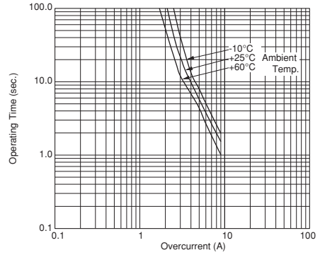
PTGL12AR0R2M1B51B0
