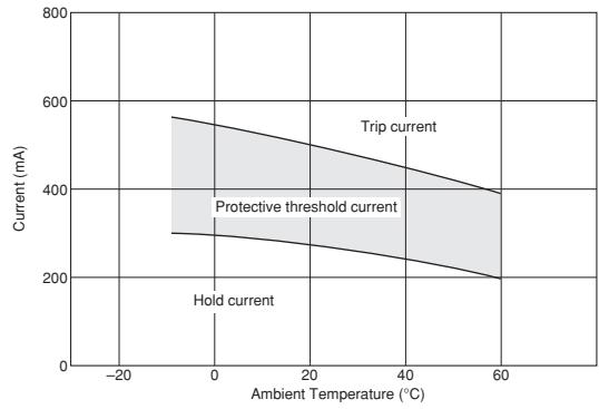
PTGL13AR100H8B72B0
