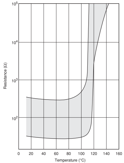
PTF_04BB222Q Type
